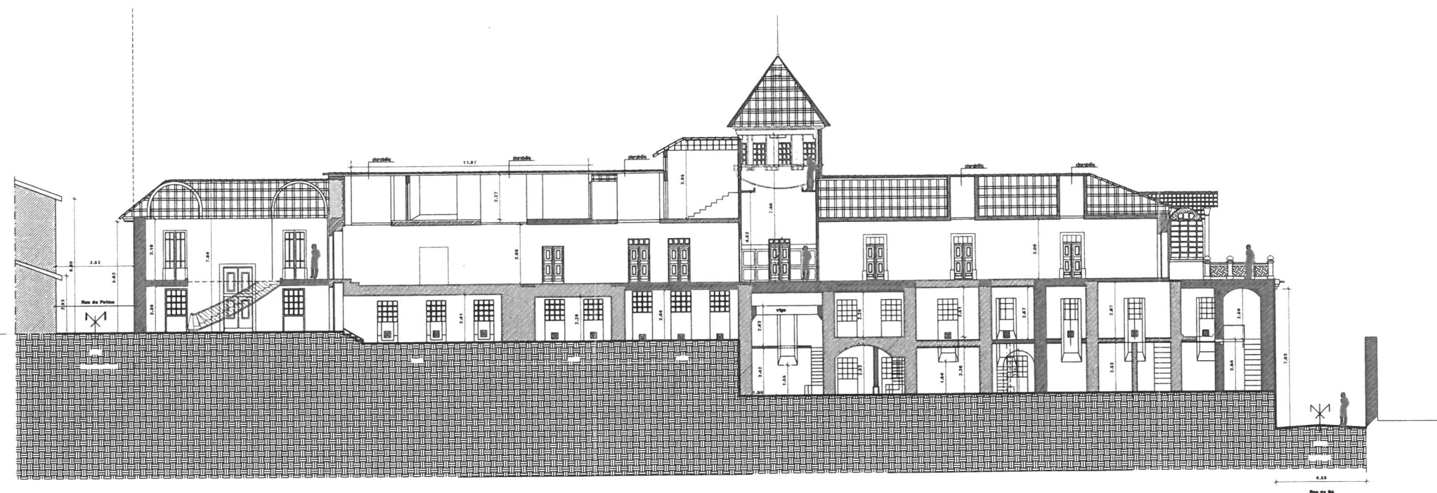
Corte 1-2 (Casa Marrocos - Edstente)
